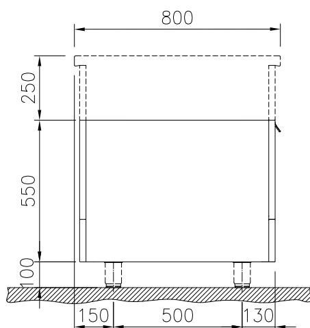
Bočna/o
